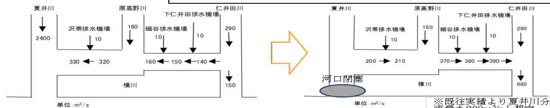
横川の流れ方向の変化 (仁井田川暫定計画規模)
