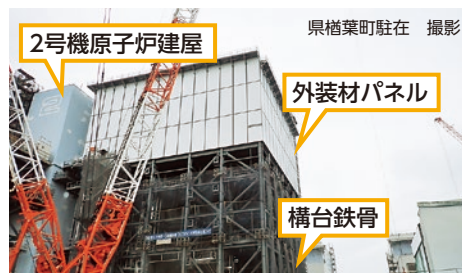
2号機の南側構台設置の様子
