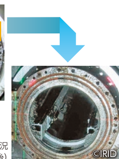
X-6 ペネの状況 (堆積物除去着手前)
