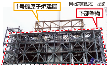
1号機の大型カバー（下部架構）設置の様子
