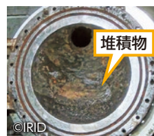
X-6 ペネの状況 (堆積物除去着手前)
