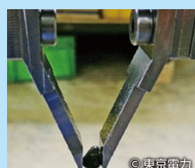
燃料デブリをつかむ先端治具（グリッパ型）
