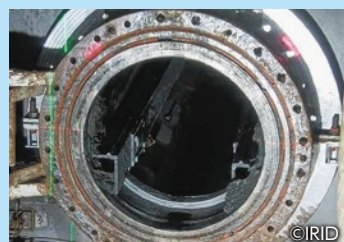
堆積物除去後の X-6 ペネ
